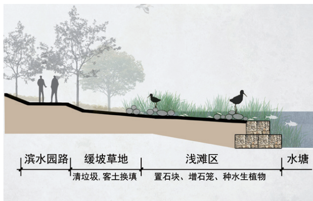
图2 生态驳岸断面示意图
